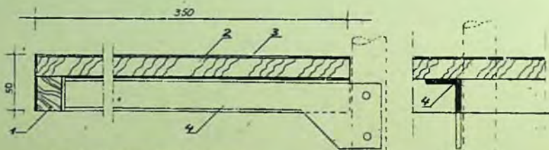
SECȚIUNE VERTICALĂ PRIN PLACĂ - MASA DEMONTABILĂ
