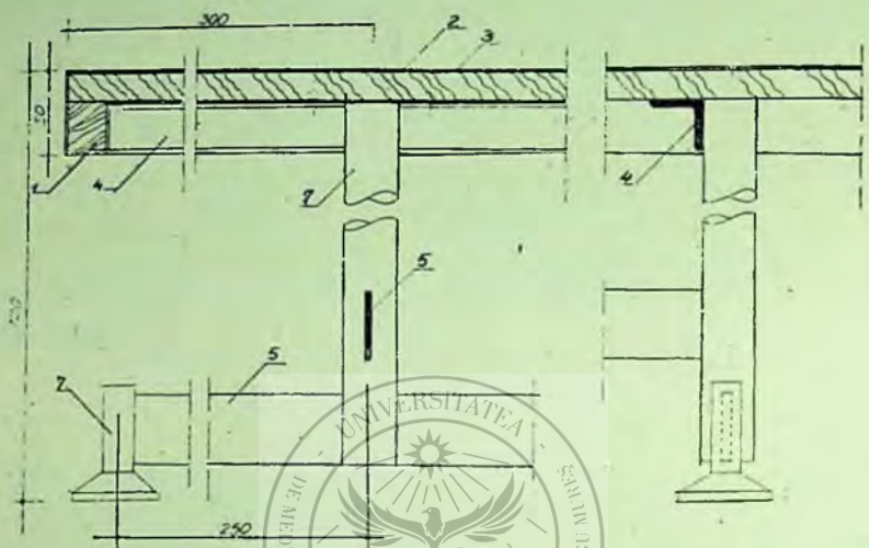
SECȚIUNI VERTICALE LA MASA
