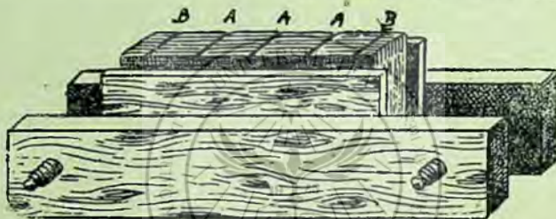
Fig. 3. — Increștarea cotorului: A = creștături de bază; B = creștături de legătură.
