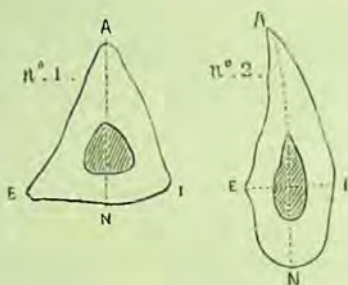
FIG. 27. — 1, coupe d'un tibia ordinaire au niveau du trou nourricier; 2, coupe au même niveau d'un tibia platycnémique; AI, face interne; AE, face externe; N, face postérieure.
